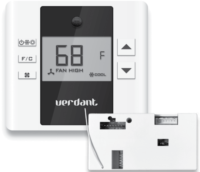
Wiring Table - 24V AC
